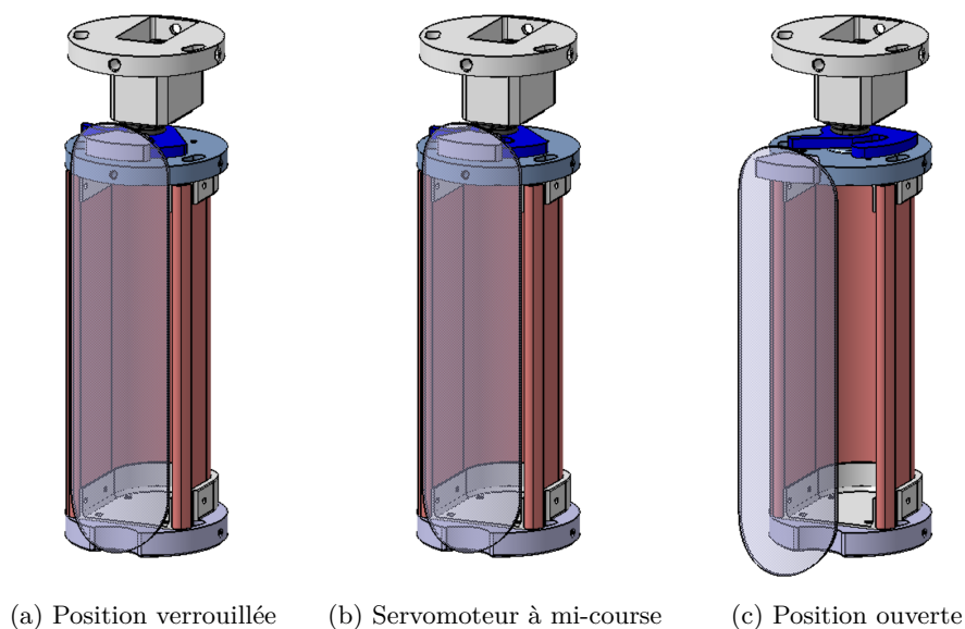
FIGURE 4.17 – Bloc parachute du second étage sur CATIA
