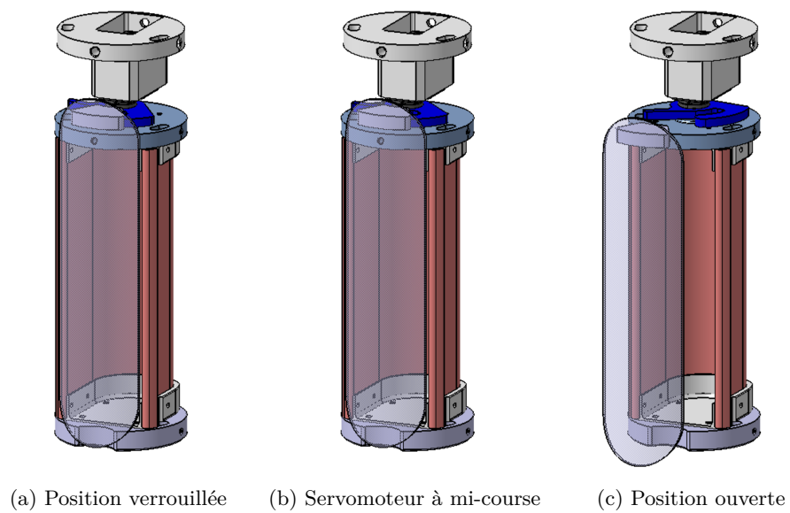
FIGURE 4.19 – Bloc parachute du second étage sur CATIA
