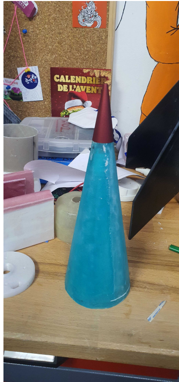
FIGURE 4.18 – Coiffe du second étage avec pointe et baromètre intégrés
