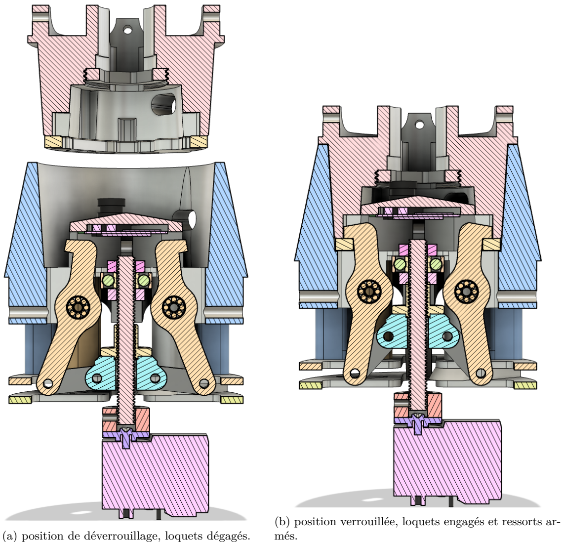
FIGURE 4.12 – Vue en coupe du mécanisme de séparation inter-étages
